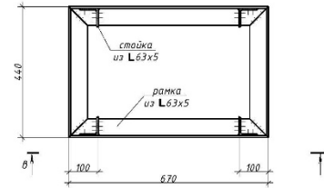
Рама для оборудования РМК-3
